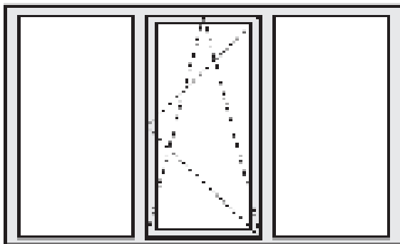
Vast / draai-kiep/ vast
