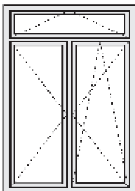
Draai/ draai-kiep met kiep bovenraam
